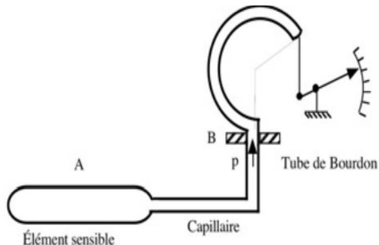
Thermomètre à gaz
