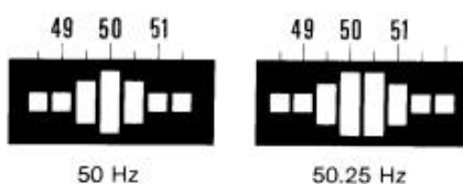
Fréquencesmètre mécanique à lamelles.
