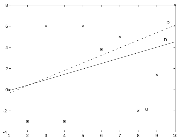
Figure B.2 : Droite de régression
