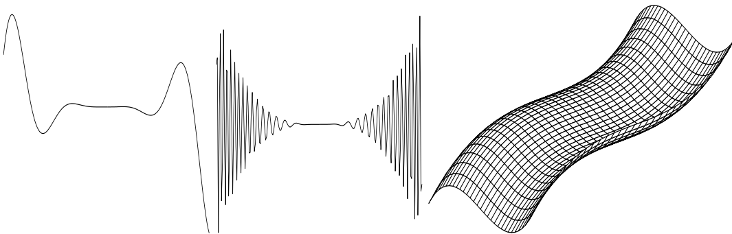
Figure 2.2 : exemples de fonctions non coercives
