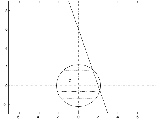
Figure 3.4 : Ensemble C des contraintes
