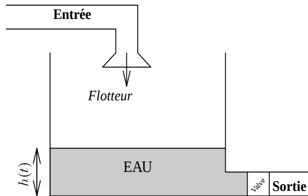
Figure 4.1. Réservoir
