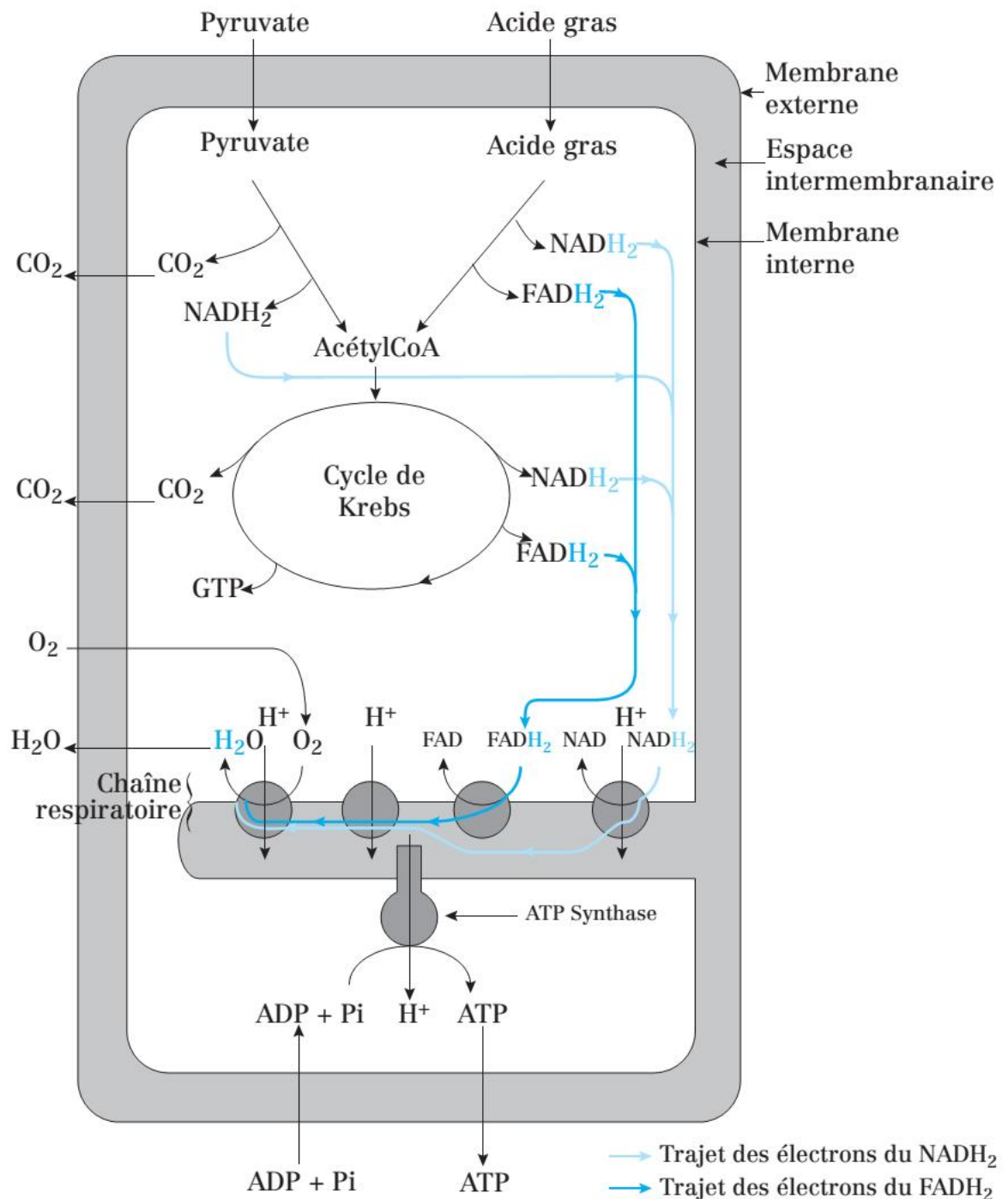
Figure 2 : Résumé des événements et acteurs conduisant à la production d'énergie dans une mitochondrie.
