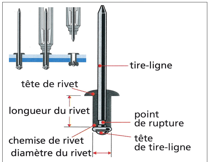
Figure 6: Principe du rivet aveugle (5)
