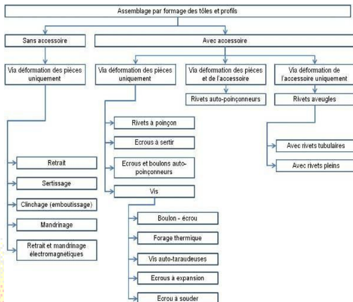
Figure 1: Aperçu des techniques d'assemblage mécanique
