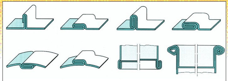
Figure 2: Exemples d'assemblages par sertissage. Un exemple connu du sertissage est l'assemblage entre le fond et le corps d'une boîte de conserve
