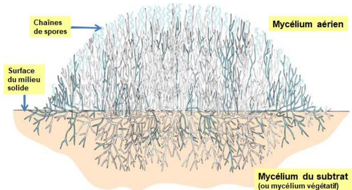
Figure 7 : Colonie d'un actinomycète poussant sur milieu solide
