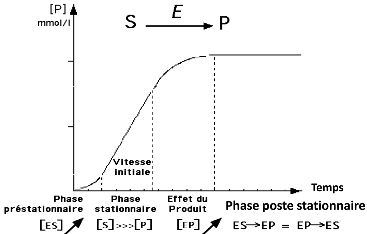
Fig. 2 Phases de la réaction enzymatique
