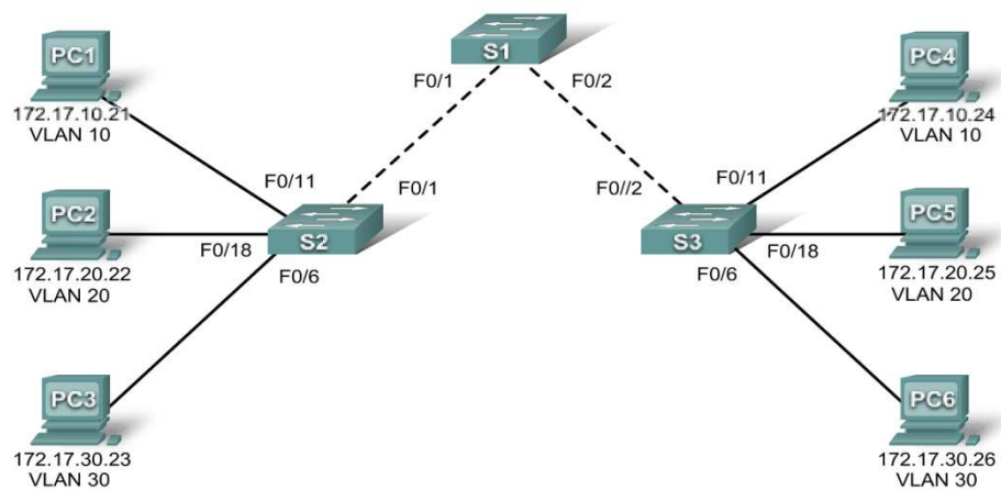
Schéma de topologie
