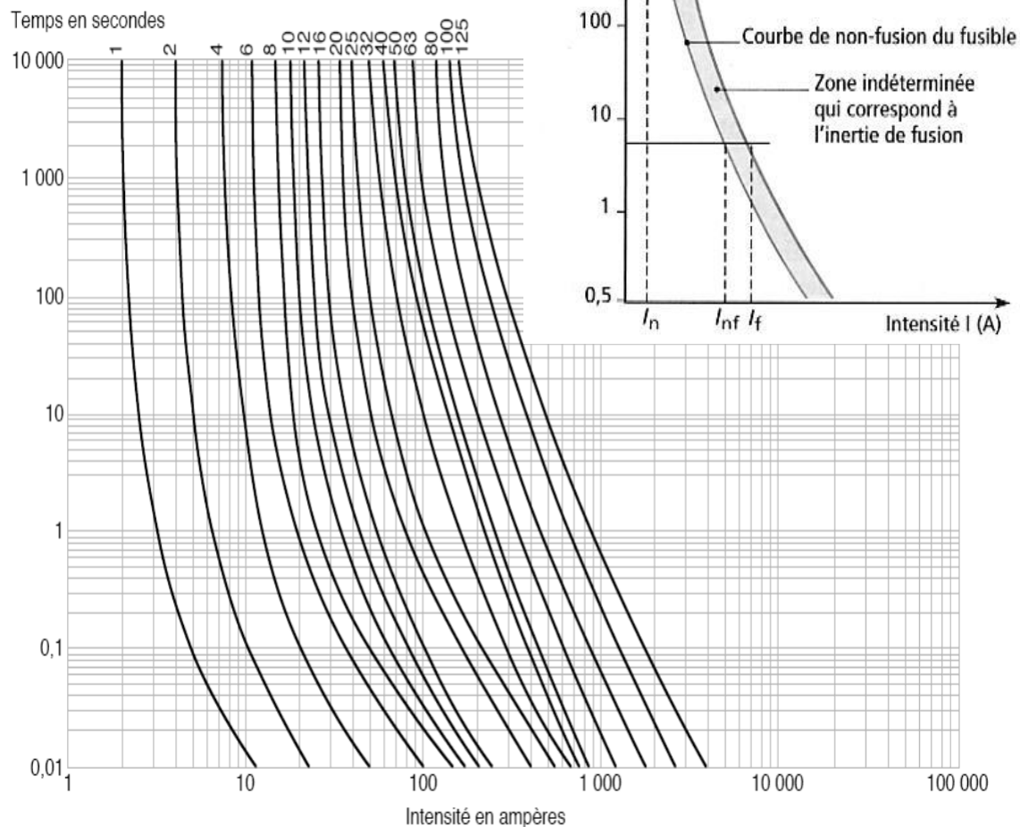
Courbes de fusion des fusibles cylindriques de classe gG.
