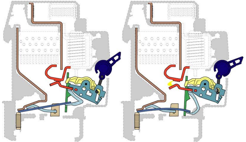
Circuit fermé
