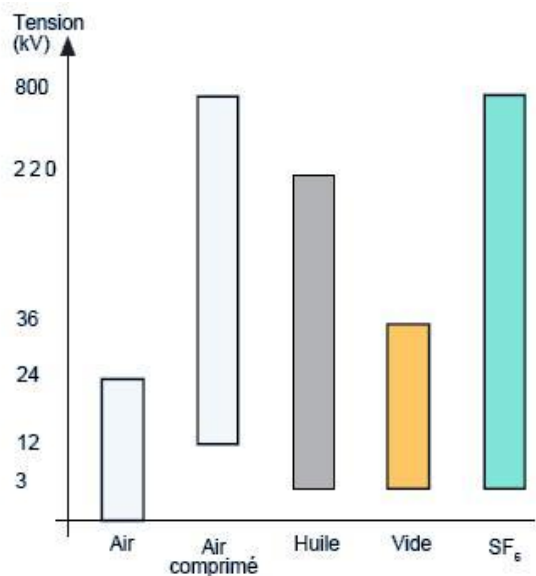
Fig.5 : Domaine d'utilisation des différents milieux de coupure
