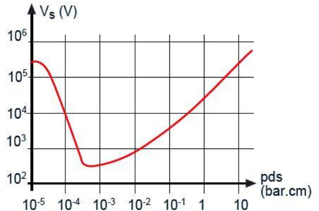
Fig.3 : La courbe de Paschen
