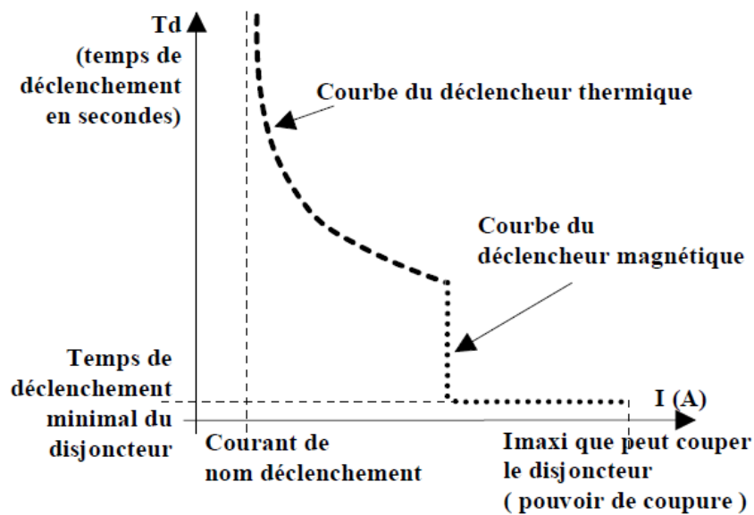
Courbe de déclenchement du disjoncteur magnétothermique
